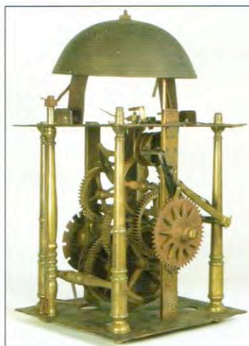
Afbeelding 5 - De voor- en linkerzijde van het uurwerk
