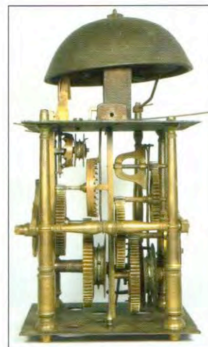
Afbeelding 6 - De rechterzijde van het uurwerk
