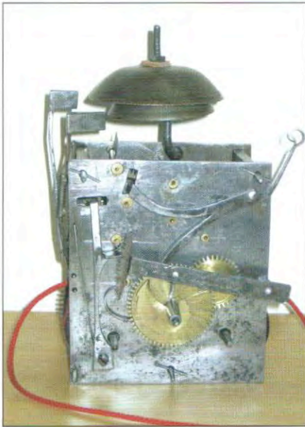
Afb. 4 - Het uurwerk bestaat uit ijzeren platines met ruwe, geklonken messing bussen.
