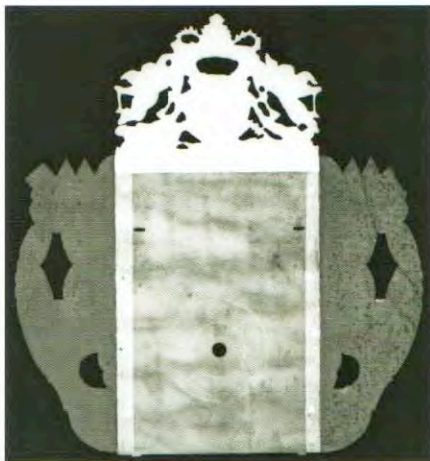
Afbeelding 2 - Röntgenfoto van de wijzerplaat
