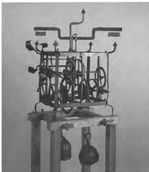
Foto 1 - Torenuurwerk, ca. 1520 (Collectie MNU)
