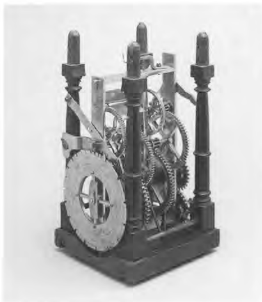
Foto 4a - Uurwerk Zaanse armeluis klok, 1717 (Collectie MNU)
