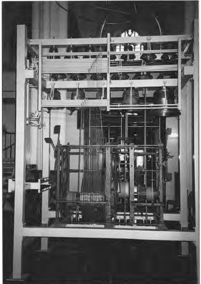
Foto 7 - De gemonteerde klok met carillon opgesteld in het Nationaal Museum van Speelklok tot Pierement.
