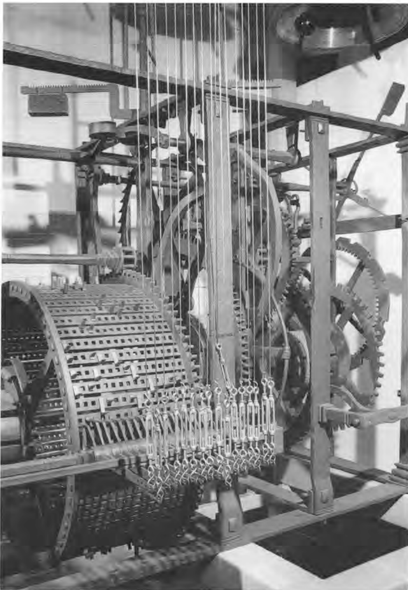
Foto 6 - Detail trommelspeelwerk met klavier. (Foto: Nationaal Museum van Speelklok tot Pierement)
