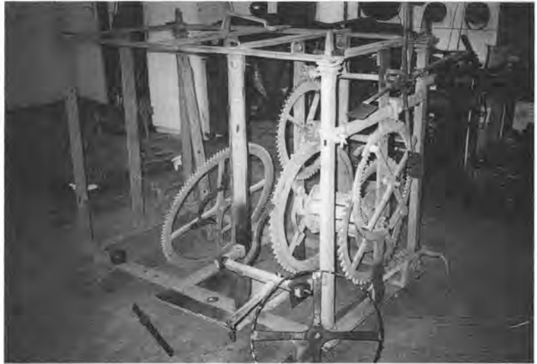
Foto 2 - De toestand na het schoonmaken van de kooi, de raderen etc.
